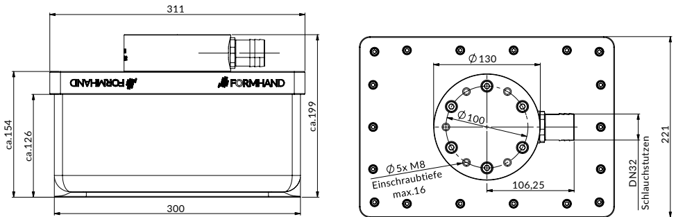
Abbildung: Ansichten des FORMHAND-Modul FH-E3020 in der Standardkonfiguration Illustration: Views of FORMHAND-Module FH-E3020 in standard configuration
