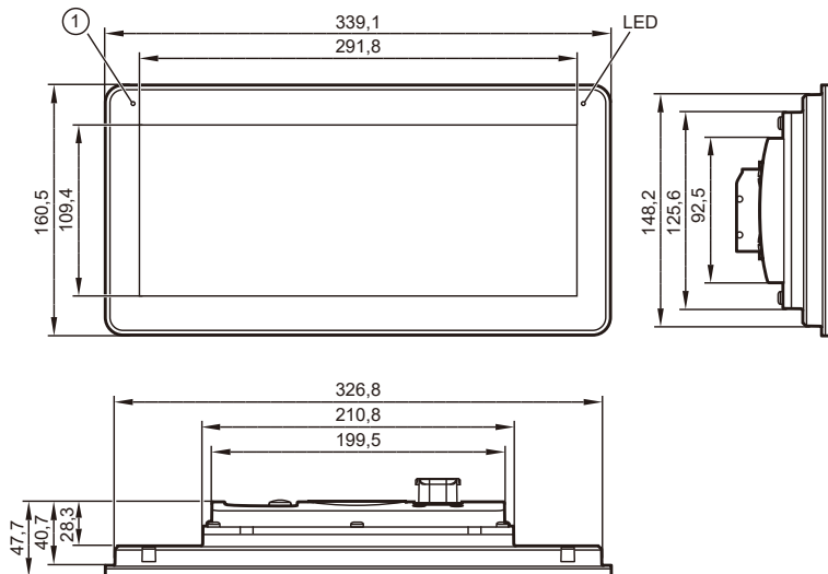
1: 光センサー
