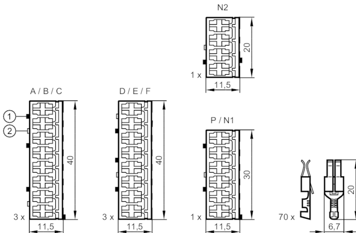
Abbildung zeigt Kontakt-Gehäuse mit geschlossenen Deckeln Ansicht auf Kontakt-Einsteckseite
