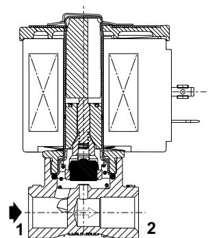
NO-Funktion
