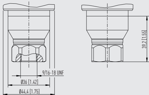
Gewindeanschluss 9/16 - 18 UNF
