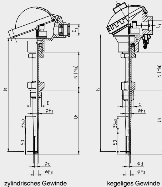
zylindrisches Gewinde
