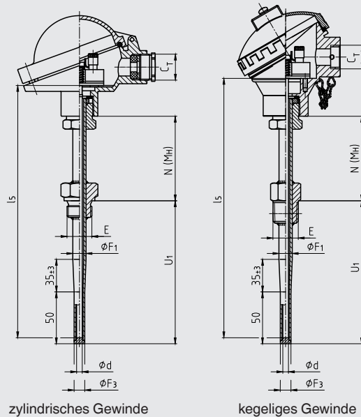
zylindrisches Gewinde
