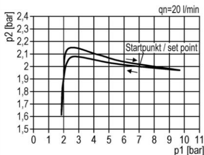
Hysterese
