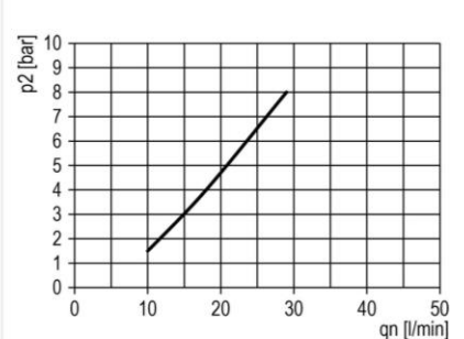
Öleransprechgrenze
