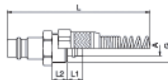
Nippel für Schlauch mit Überwurfmutter, Knickschutzfeder
