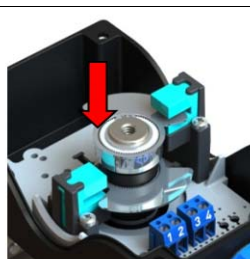
Abb. 3: Schlitz-Betätiger
