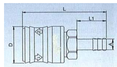
Schlauchtülle
