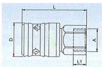
Innengewinde
