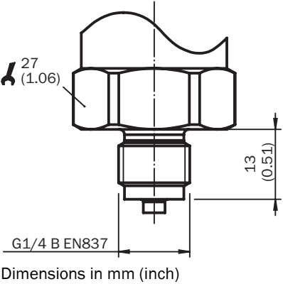
Dimensional drawing G \frac{1}{4} B (EN 837)
