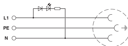
Schaltplan
