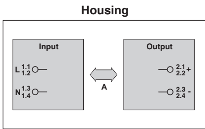
Schemazeichnung
