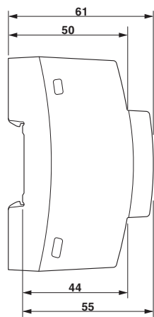
Maßzeichnung
