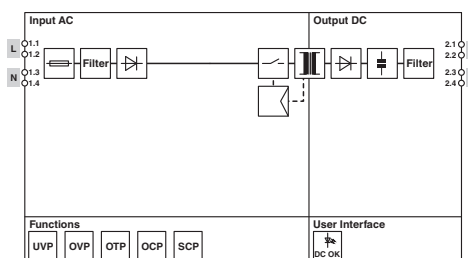
Blockschaltbild
