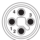
Polbild Stecker M12, 4-polig, T-kodiert, Ansicht Steckerseite
