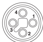
Polbild M12-Buchse, 4-polig, T-kodiert, Ansicht Buchsenseite
