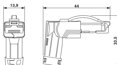
RJ45-Steckverbinder, IP20, gewinkelt
