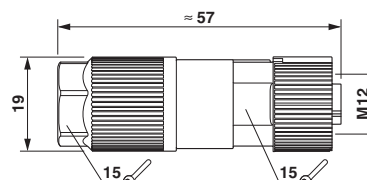
Maßzeichnung
