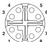
Polbild M12-Buchse, 8-polig, Ansicht Buchsen-seite
