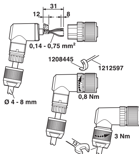
Funktionszeichnung
