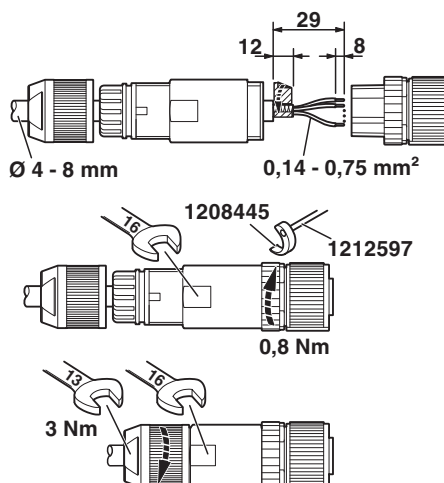
Funktionszeichnung
