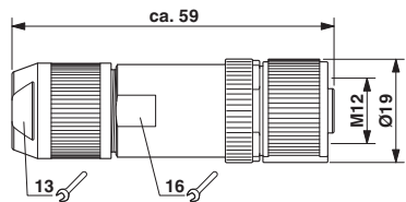
Maßzeichnung
