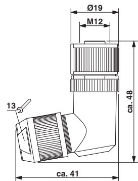
Maßzeichnung
