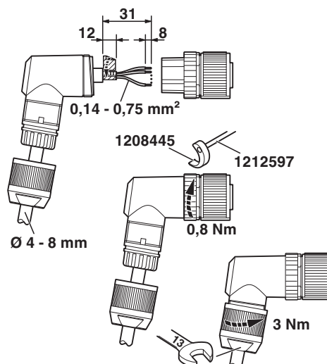
Funktionszeichnung
