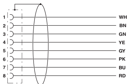
Schaltplan
