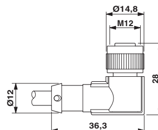
Maßzeichnung
