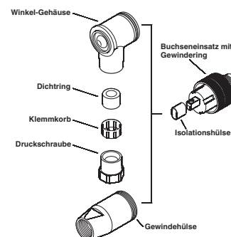
Stecker/Buchse M12
