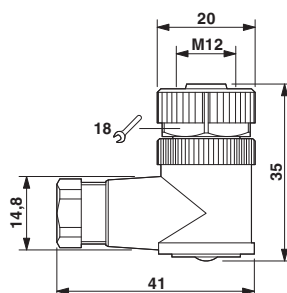
Buchse M12 x 1, gewinkelt
