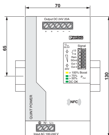
Maßzeichnung
