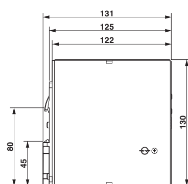
Maßzeichnung
