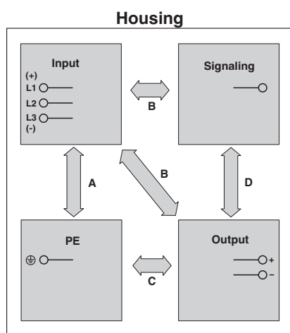
Blockschaltbild
