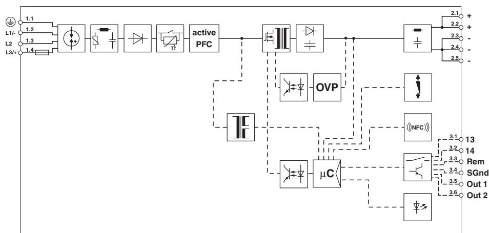
Blockschaltbild
