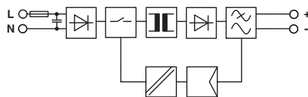
Blockschaltbild
