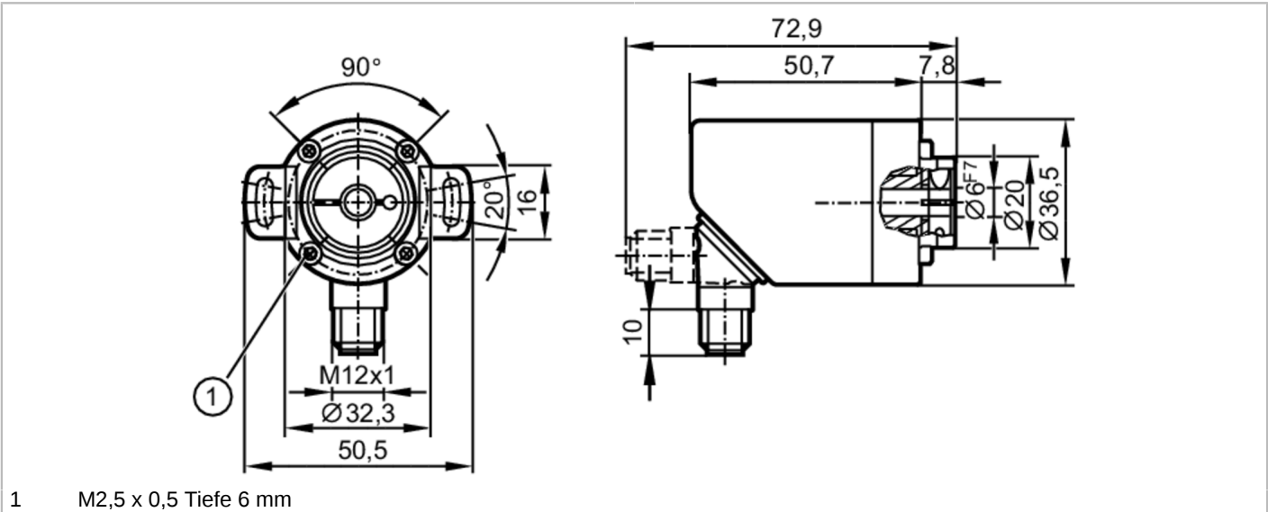
1 M2,5 x 0,5 Tiefe 6 mm
