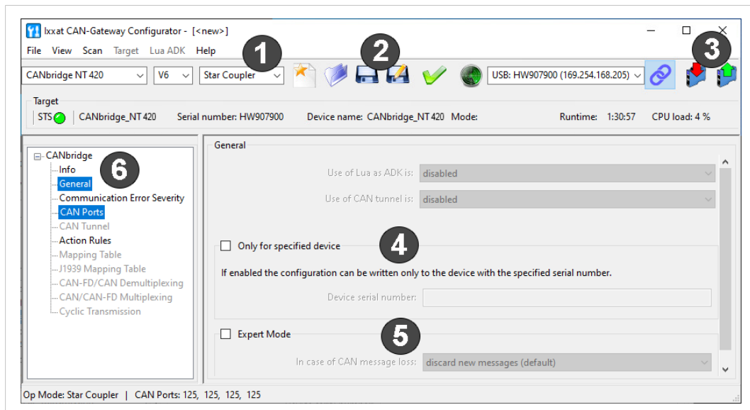
Fig. 4 Repeater-Konfiguration
