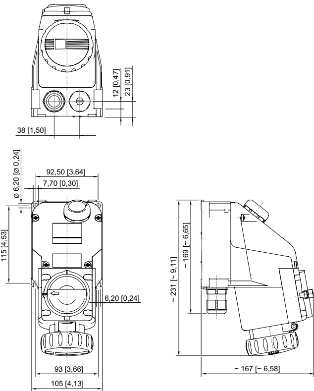
Reparatursteckdose 3-polig
