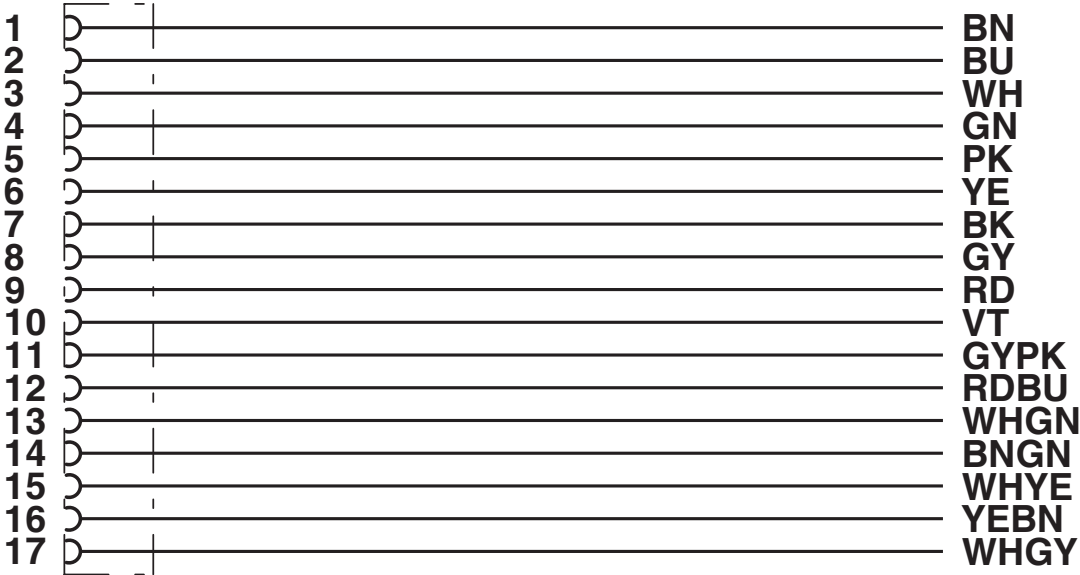
Schaltplan
