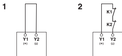
Bild 14 Anschlussvarianten Startkreis
