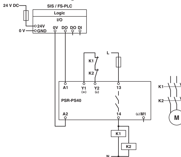
Bild 15 High-Demand-Applikation mit fehlersicherer Steuerung
