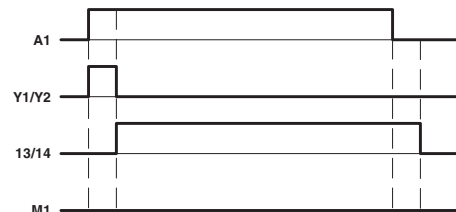
Zeitdiagramm automatischer Start
