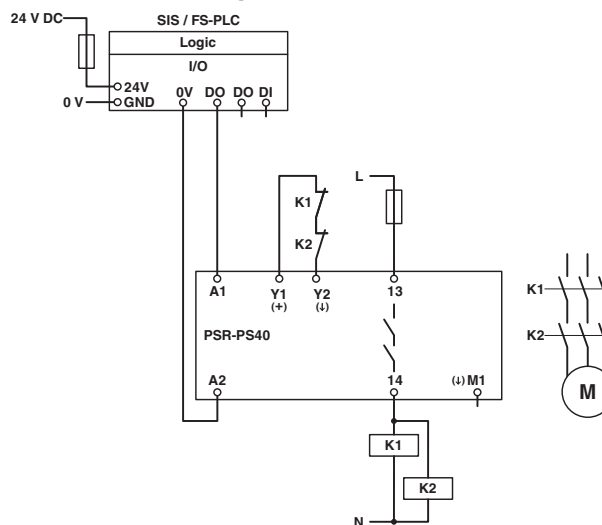
Bild 16 Low-Demand-Applikation mit fehlersicherer Steuerung
