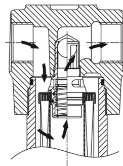
Filtrationsbetrieb
