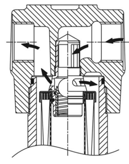
Reversierbetrieb
