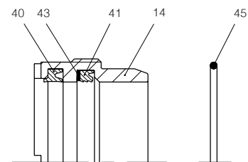
Dichtungsbüchse mit Dichtungen
