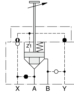
D4S...233B. mit Hubbegrenzer Steuerölzulauf X = extern
