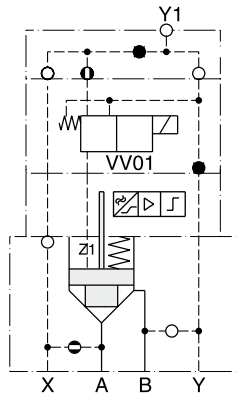
D4S...123A. BC } mit Stellungsüberwachung BE }
