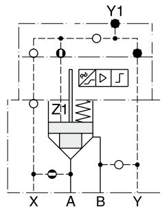
D4S...113A.BA (mit Stellungsüberwachung)
