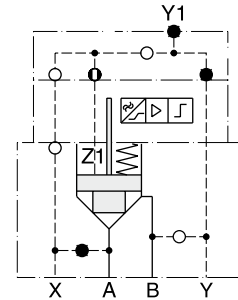
D4S...213A.BA (mit Stellungsüberwachung)
