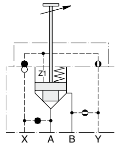
D4S...D434. mit Hubbegrenzer Steuerölzulauf Y = intern von B
