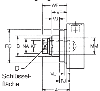
Kolbenstangenende Code 5 & 9 – Befestigungsart JJ
