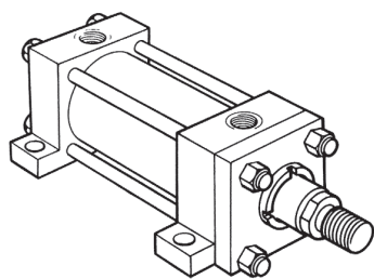
Befestigungsart C Fußbefestigung ISO-MS2 DIN-MS2
