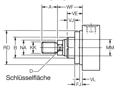
Kolbenstangenende Code 5 & 9 – Befestigungsart JJ
