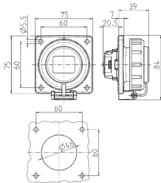
Zeichnung 1 MB 628 Maße in mm
