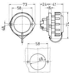
Zeichnung 1 MB 301 Maße in mm
