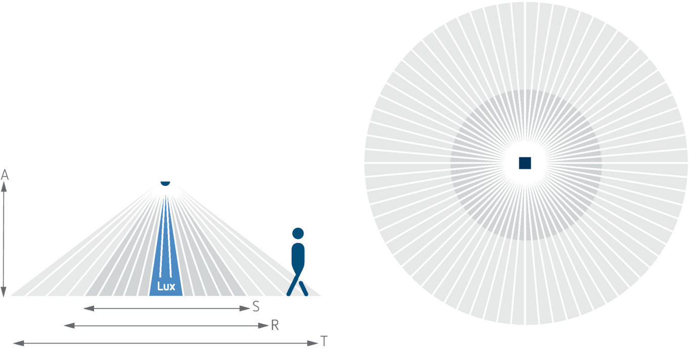
Erfassungsbereich nach Sensnorm IEC 63180
