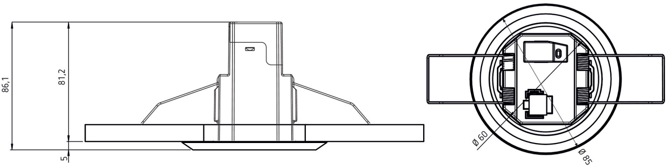
Maßzeichnungen
