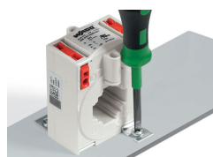
Montage auf Montageplatte
