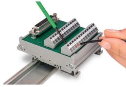
Leiter anschließen – Betätigung rechtwinklig zur Leitereinführung..
