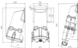
Zeichnung 1 MB 637 Maße in mm
