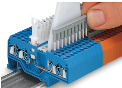
Brücken von Trennklemmen mit Frontverdrahtung mit Brückungskämmen unter Zuhilfenahme eines 10-fach-Betätigungs­werkzeuges
