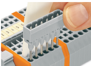
Einsetzen der Stiftleiste mit Mehrfach-Betätigungs­werkzeug
