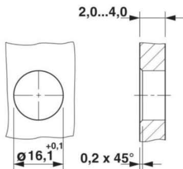
Maßzeichnung
