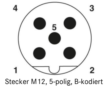
Schemazeichnung
