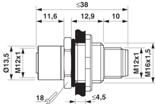
Maßzeichnung
