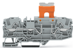
Trennstecker (2006-401) in Basisklemme (2006-1661) in Parkstellung gesteckt
