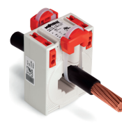
Montage mit Schnellbefestigungsadapter 855-9910
