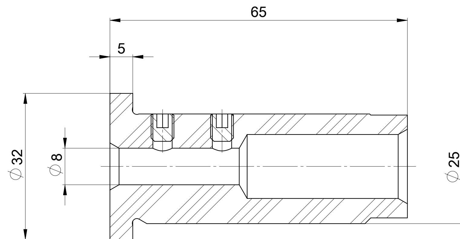
SEZIONE A-A
